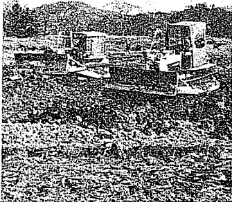
工場敷地の造成工事
