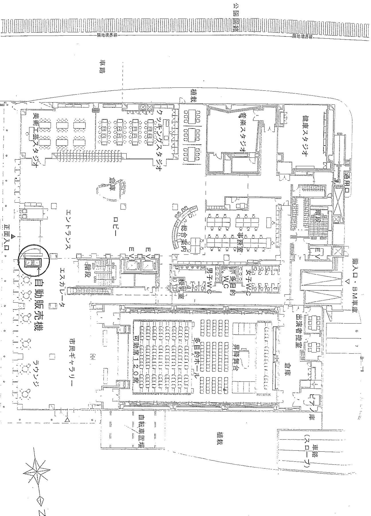
1階平面図
