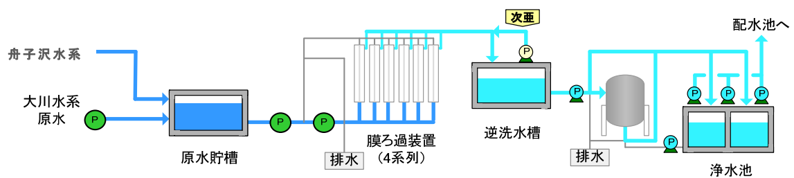
図 1.3-4 大戸浄水場処理フロー
