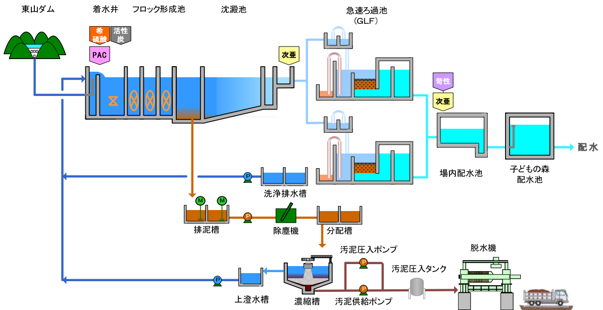
図 1.3-2 東山浄水場処理フロー
