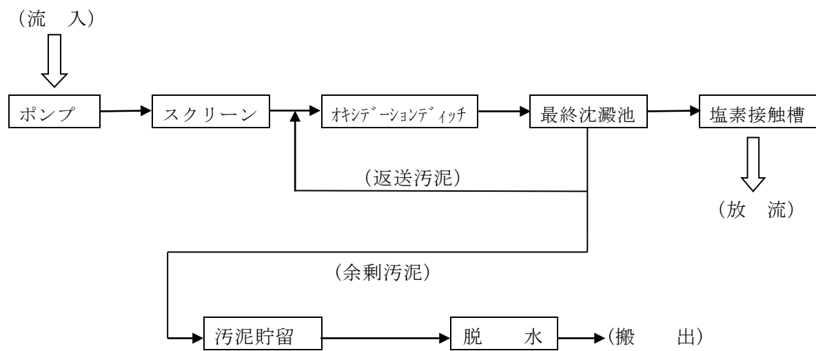
【添付図 2】 北会津北部浄化センターの処理フロー図
