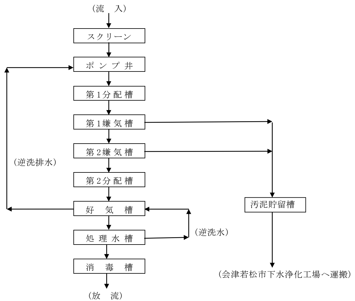
【添付図 3】 河東浄化センターの処理フロー図
