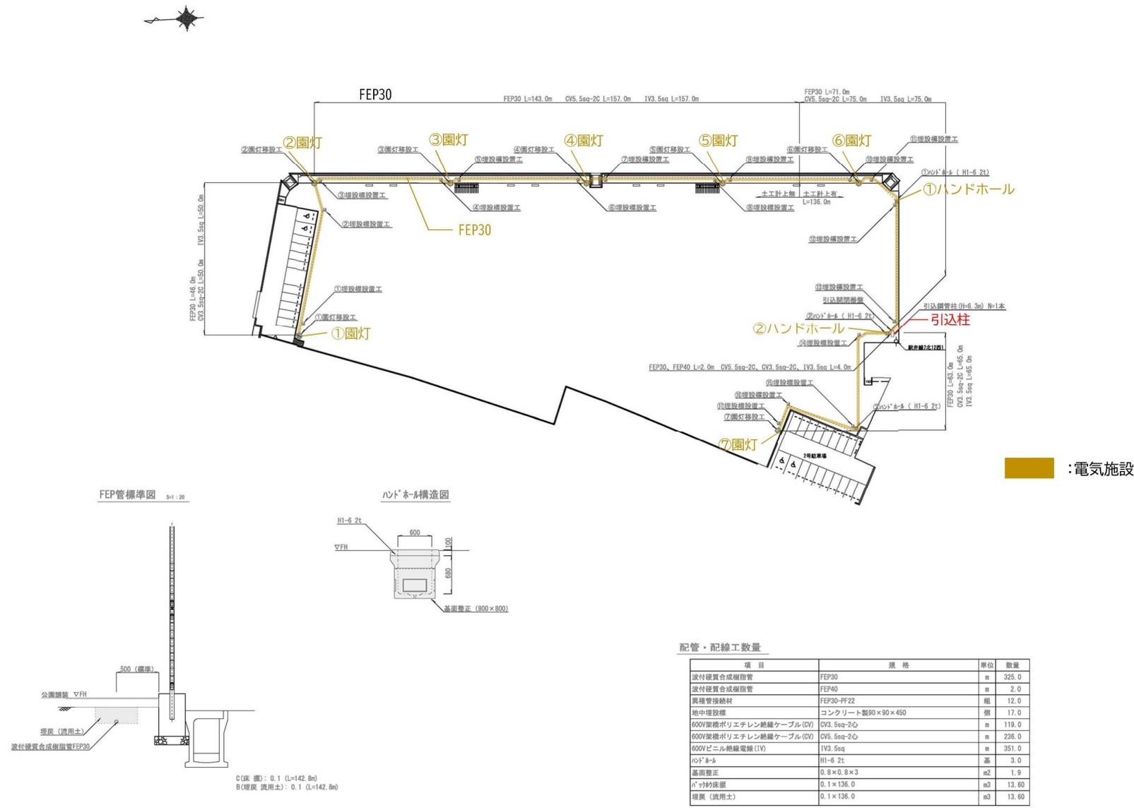
図 2-3 扇町1号公園 電気施設現況
