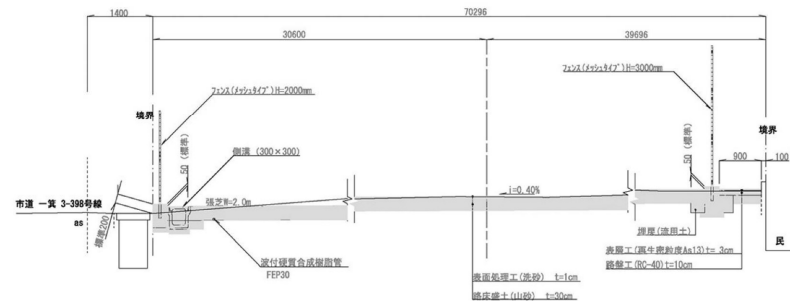
図 2-2 扇町1号公園 給水施設現況
