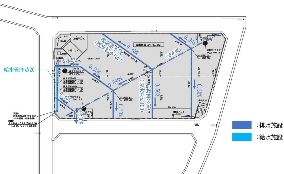
図 2-8 扇町5号公園 給排水施設現況
