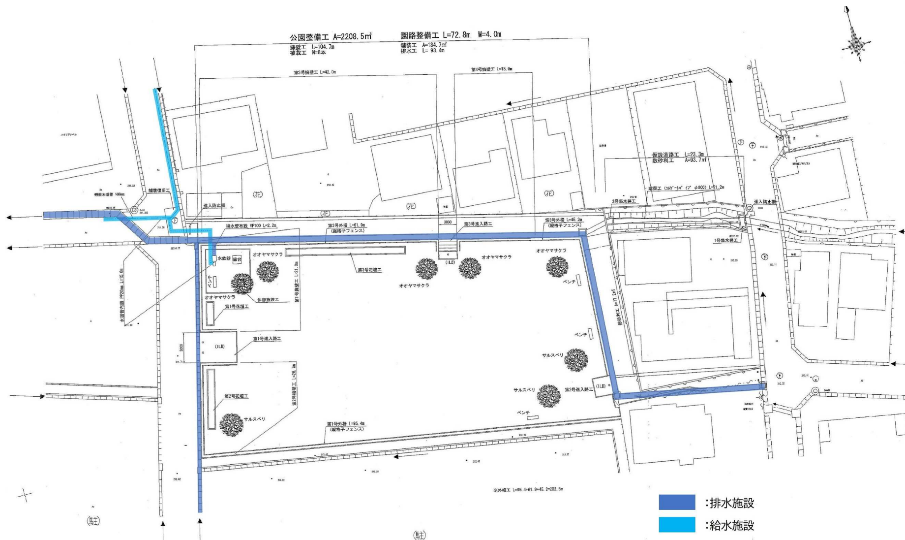
図 2-5 扇町2号公園 給排水施設現況
