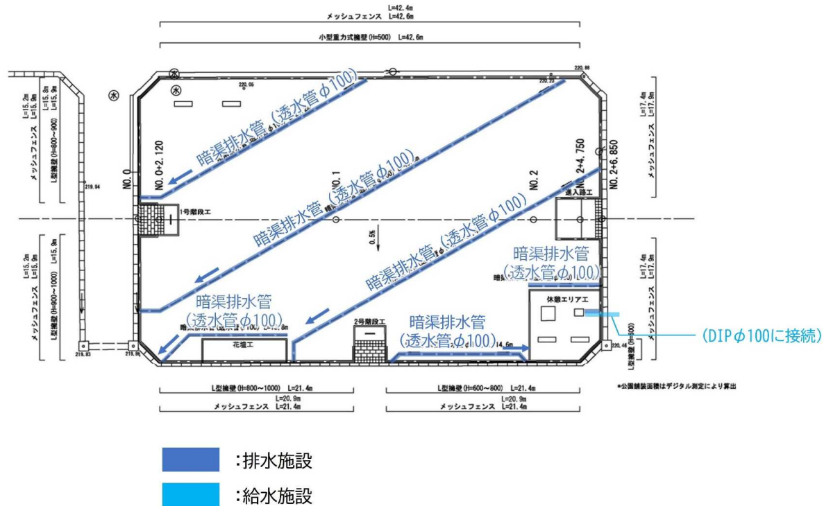
図 2-9 扇町6号公園 給排水施設現況
