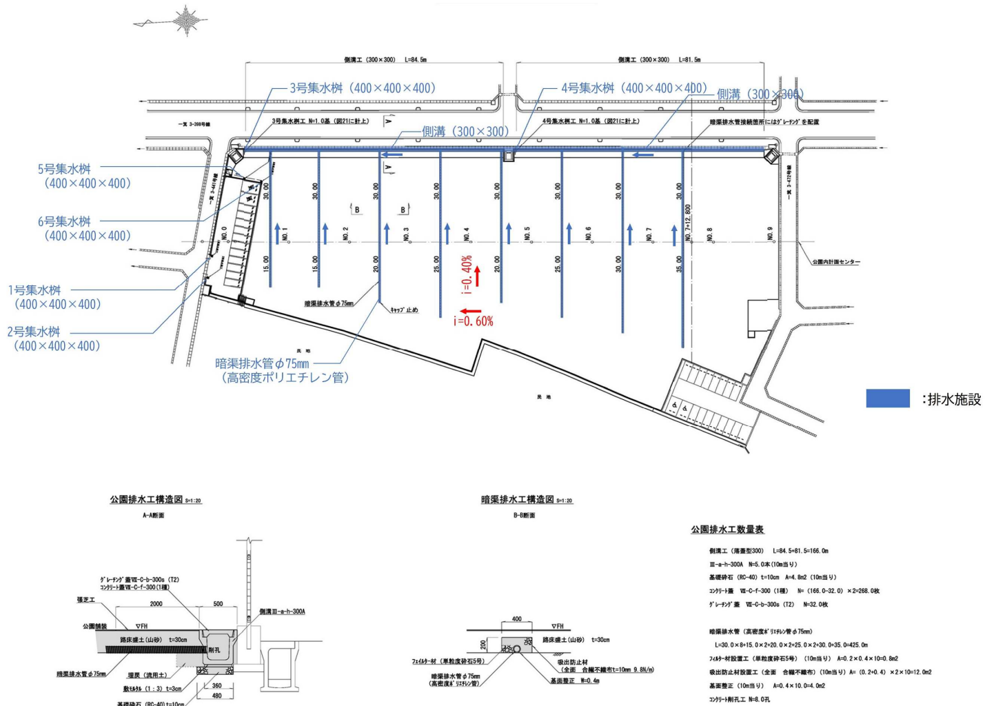
図 2-1 扇町1号公園 排水施設現況
