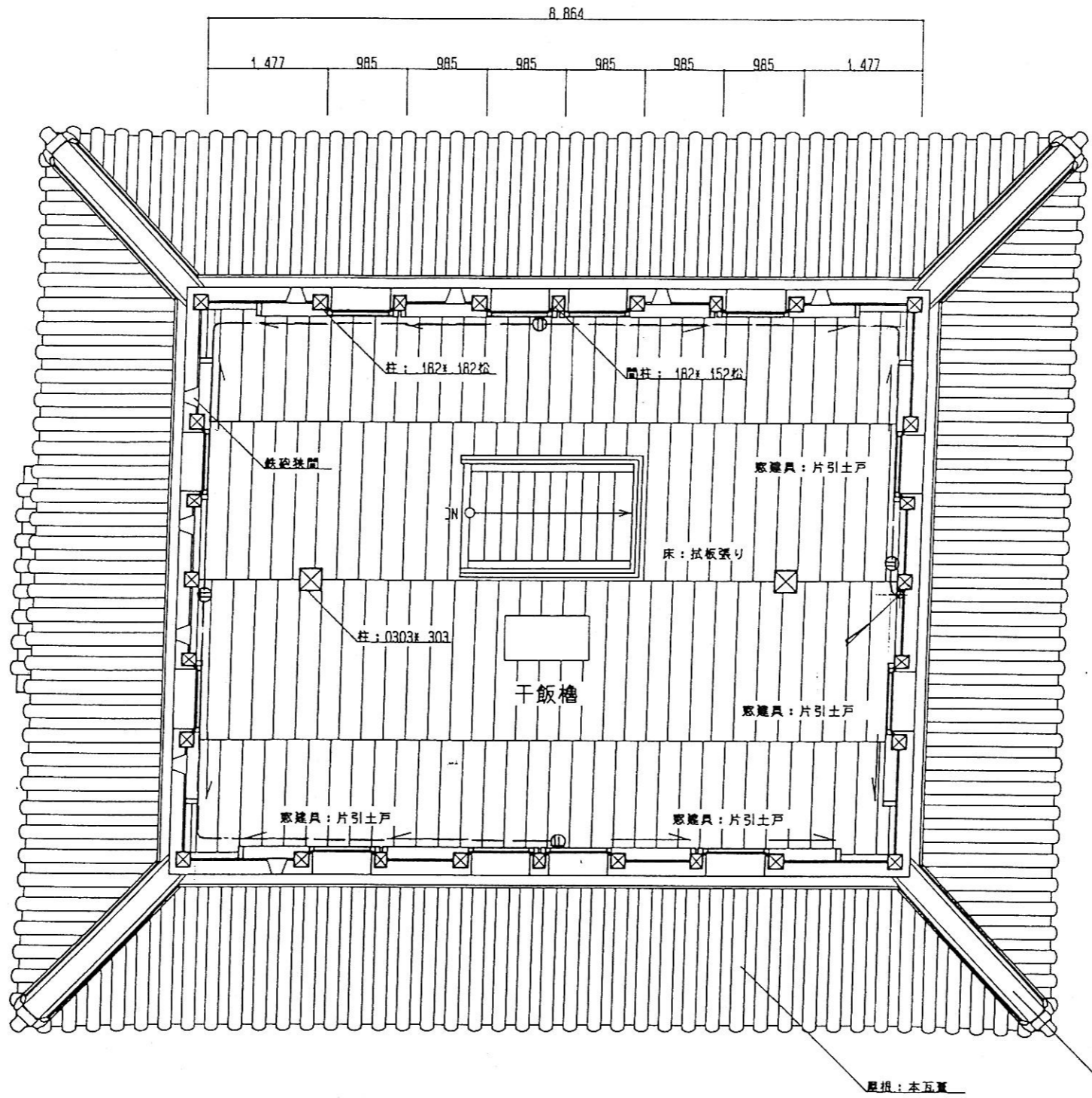
二階平面図 S: 1/50
