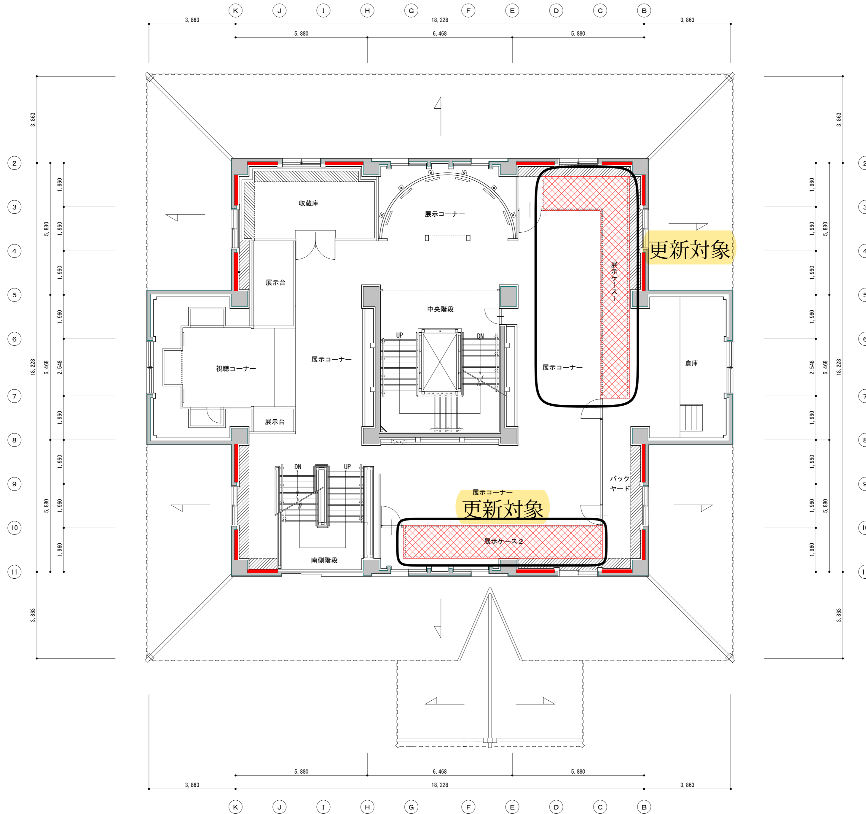
2階平面図 S=1/100
