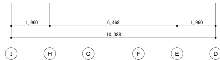
地下1階平面図 S=1/100
