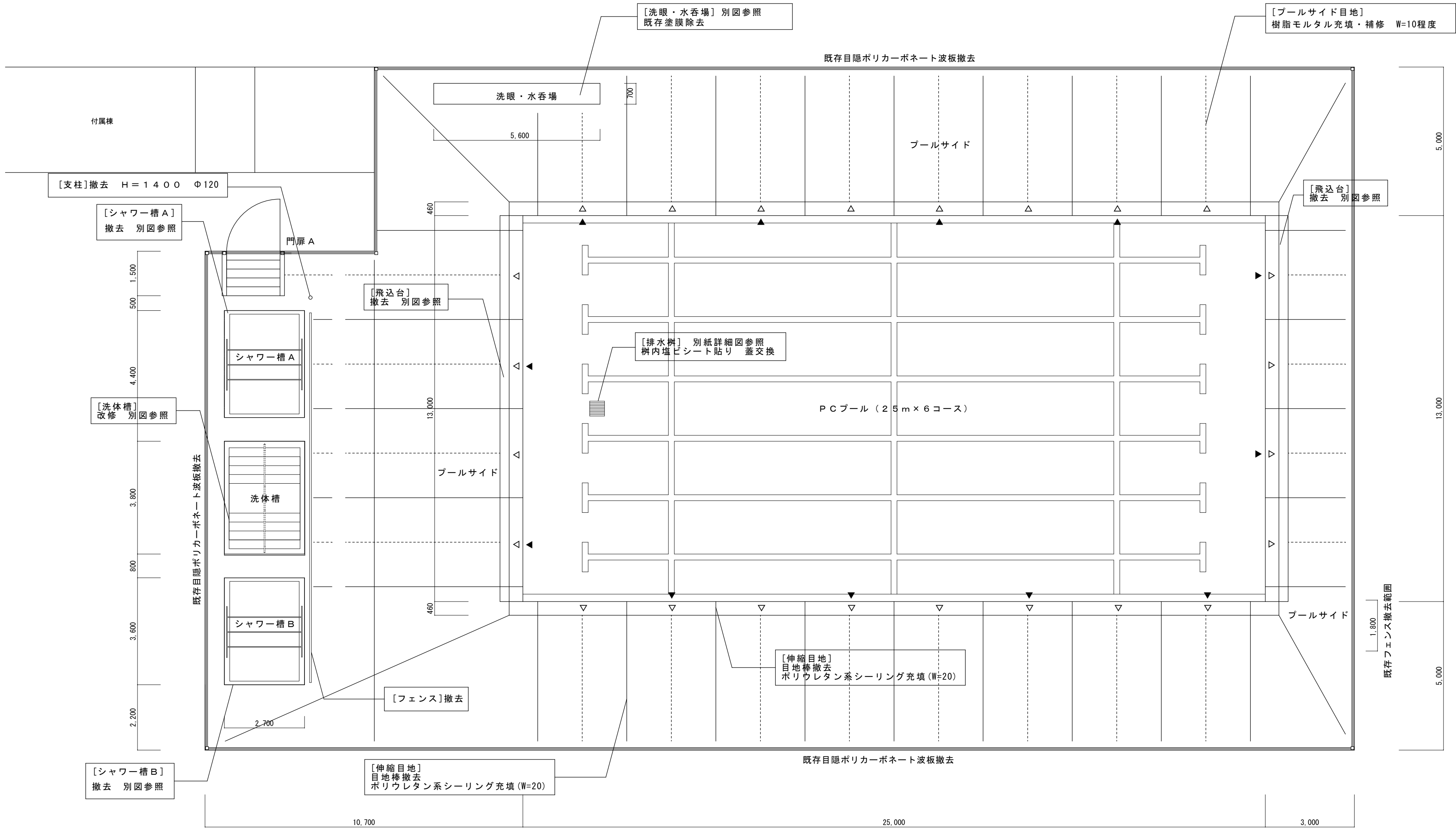
改修前平面図 S=1/100
