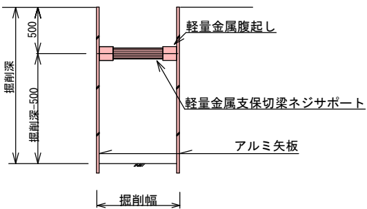
アルミ矢板断面図
