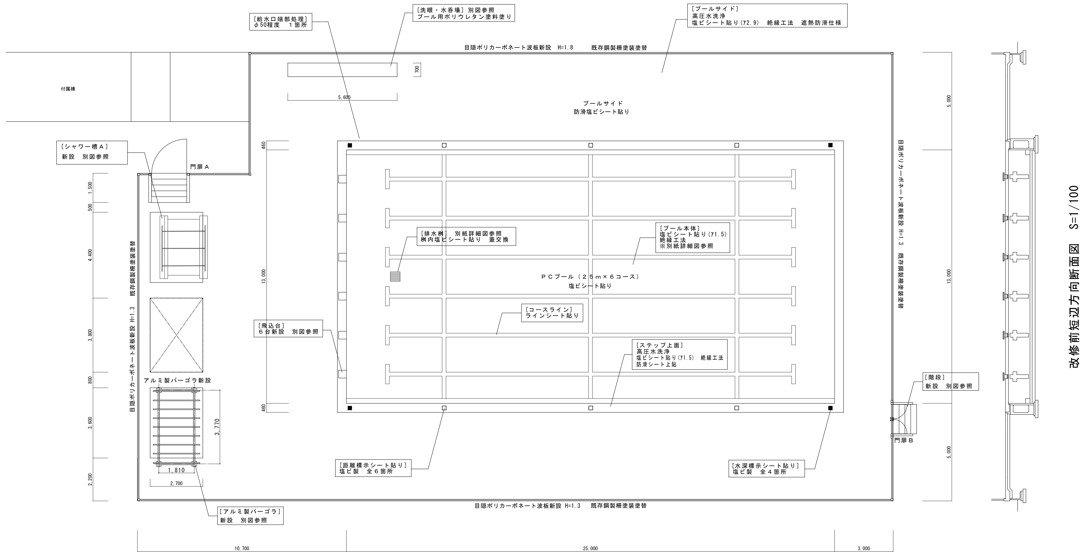
改修後平面図 S=1/100
