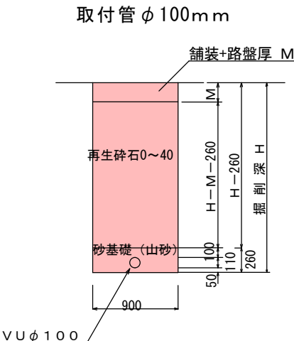
埋戻工標準断面図
