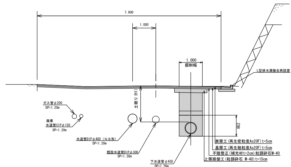
A-A'断面
