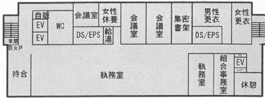
5階平面図
