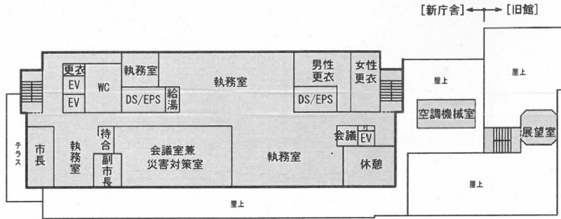
4階平面図
