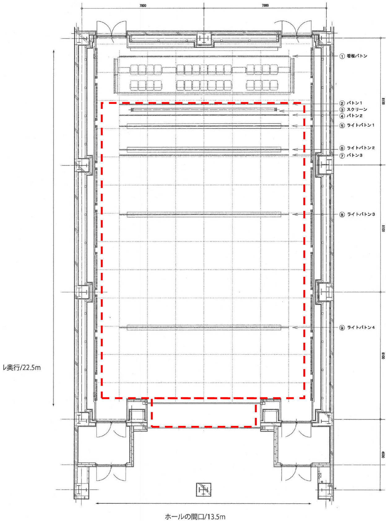
稽古堂/多目的ホール平面図
