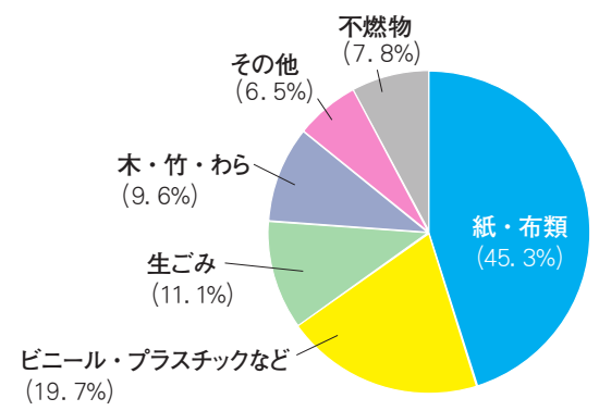
燃やせるごみの分析結果(R2年度)
