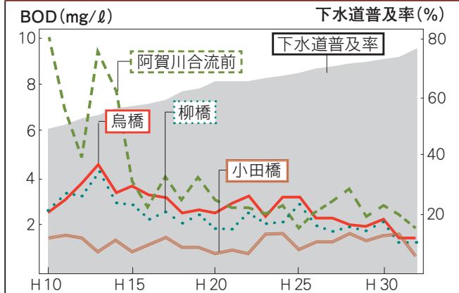
湯川の水質調査の結果
