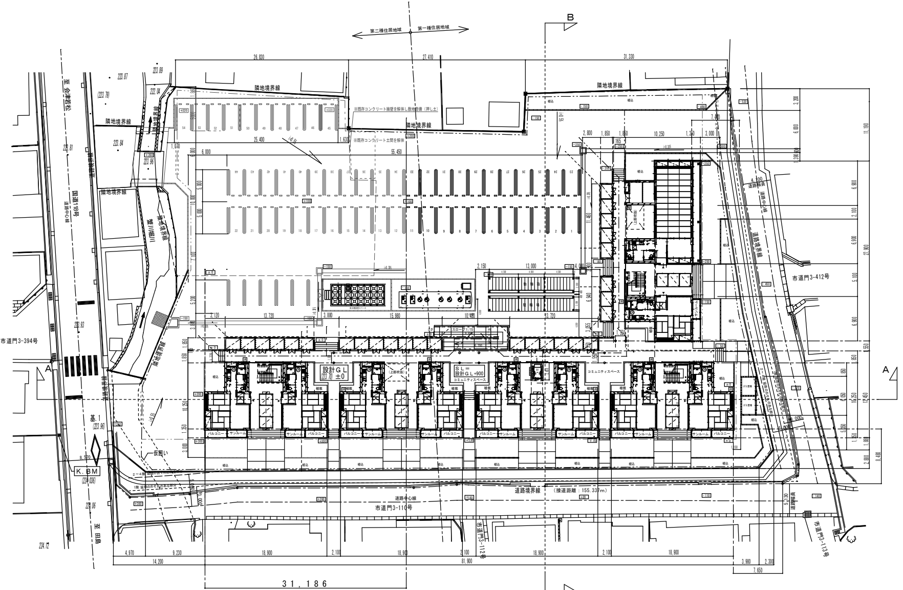
配置図 S=1/300
